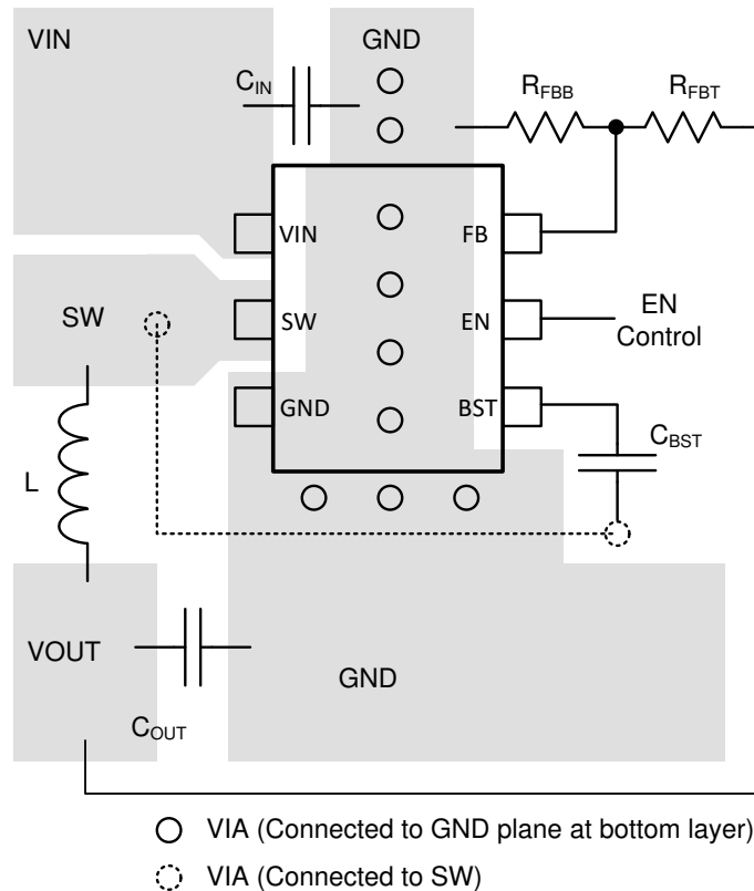
图 9-1. TPS562207 布局
