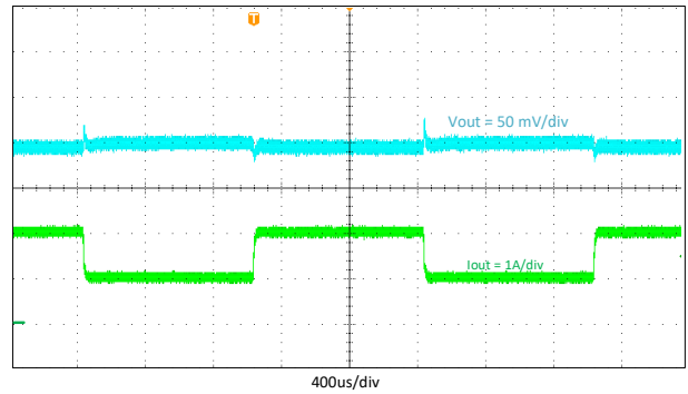
图 8-9. 瞬态响应, 1A 到 2A
