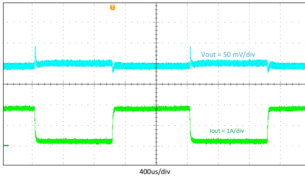
图 8-8. 瞬态响应, 0.2A 到 1.8A
