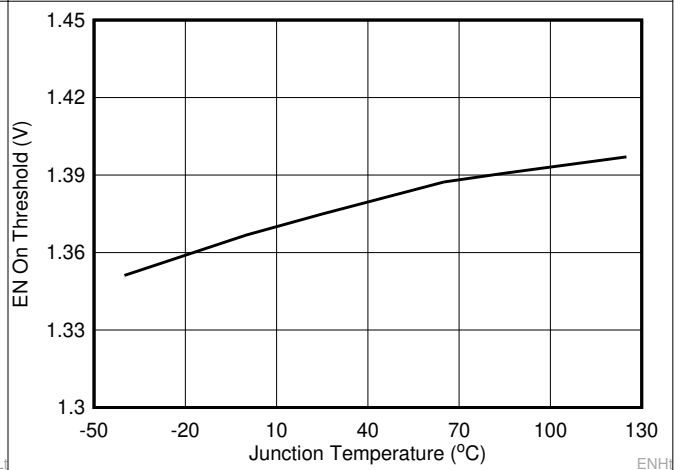
图 6-4. EN 导通阈值电压与结温间的关系
