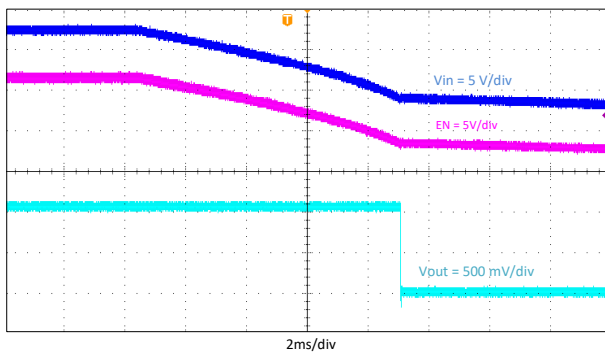
图 8-12. 相对于 VIN 的关断
