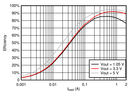
TPS562207 效率
