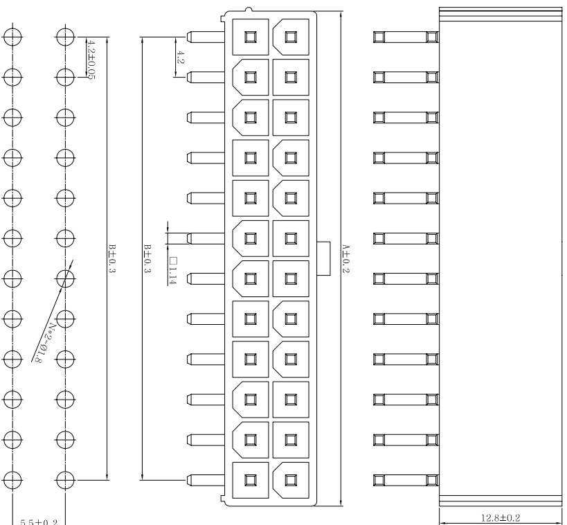
P.C.B Layout
