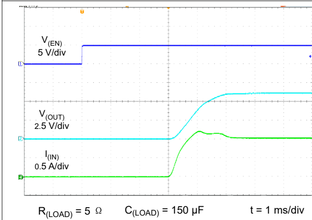
图 6-20. Turnon Response
