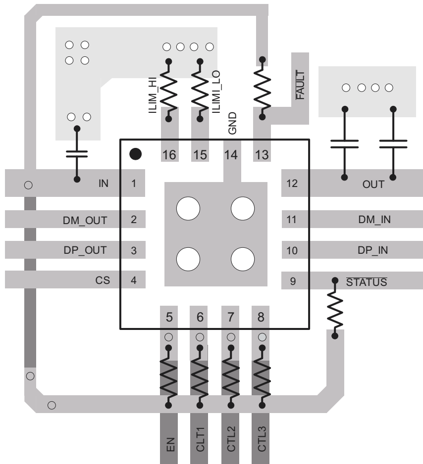
图 11-1. TPS2549-Q1 Layout Diagram
