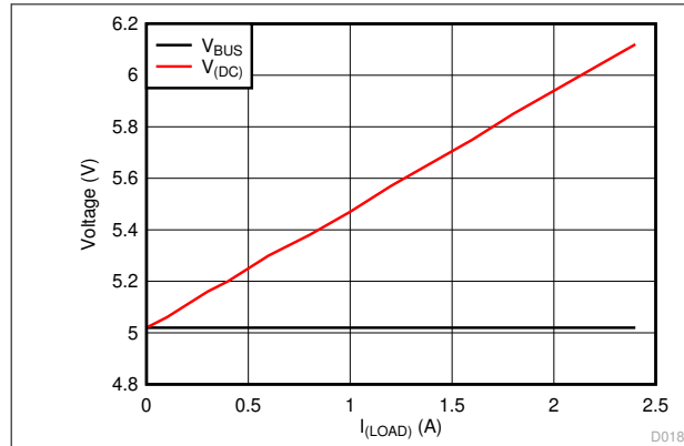
图 9-2. V_{(DC)} and V_{BUS} vs I_{(LOAD)} Output
