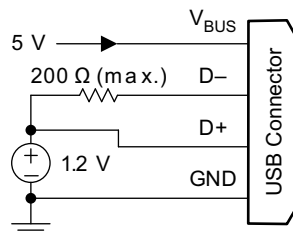
图 8-10. 1.2-V Mode
