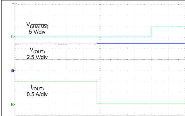
图 6-26. Hot Short
