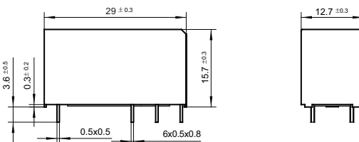
外形图
