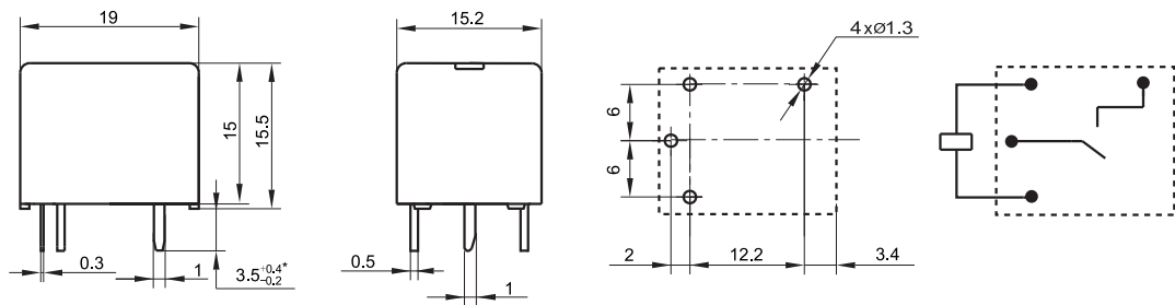
安装孔尺寸 (底视图)
