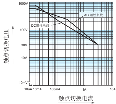
单组触点
