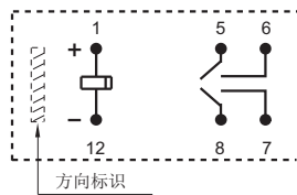
图示为释放状态
