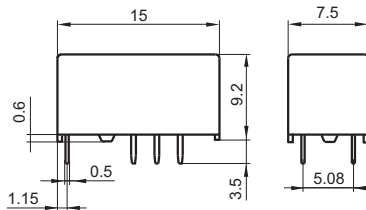
外形图
