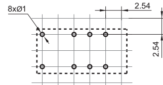
安装孔尺寸 (底视图)
