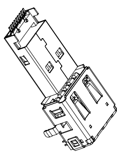
公头连接器可从正方向插入
