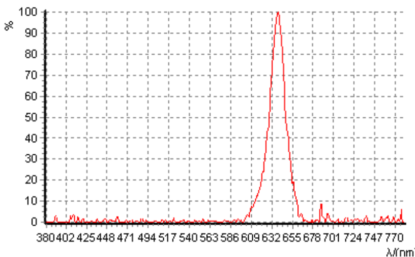
波长
