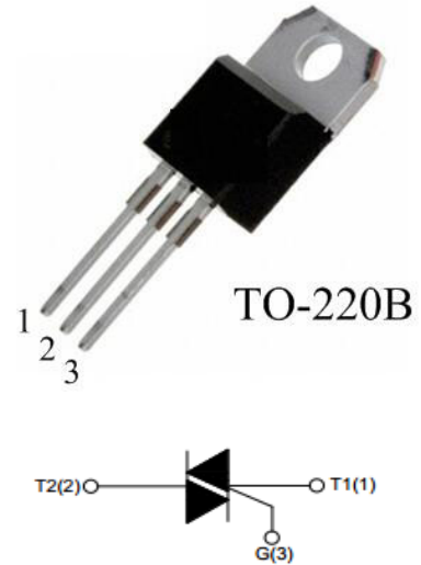
T1:主端子 T2:主端子 G:触发极
