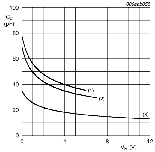
f = 1 MHz; T amb = 25 °C (1) PESD5Z6.0 (2) PESD5Z7.0 (3) PESD5Z12
