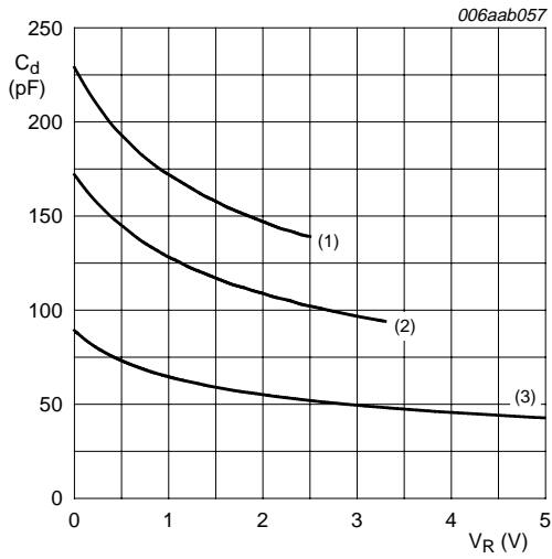
f = 1 MHz; T amb = 25 °C (1) PESD5Z2.5 (2) PESD5Z3.3 (3) PESD5Z5.0
