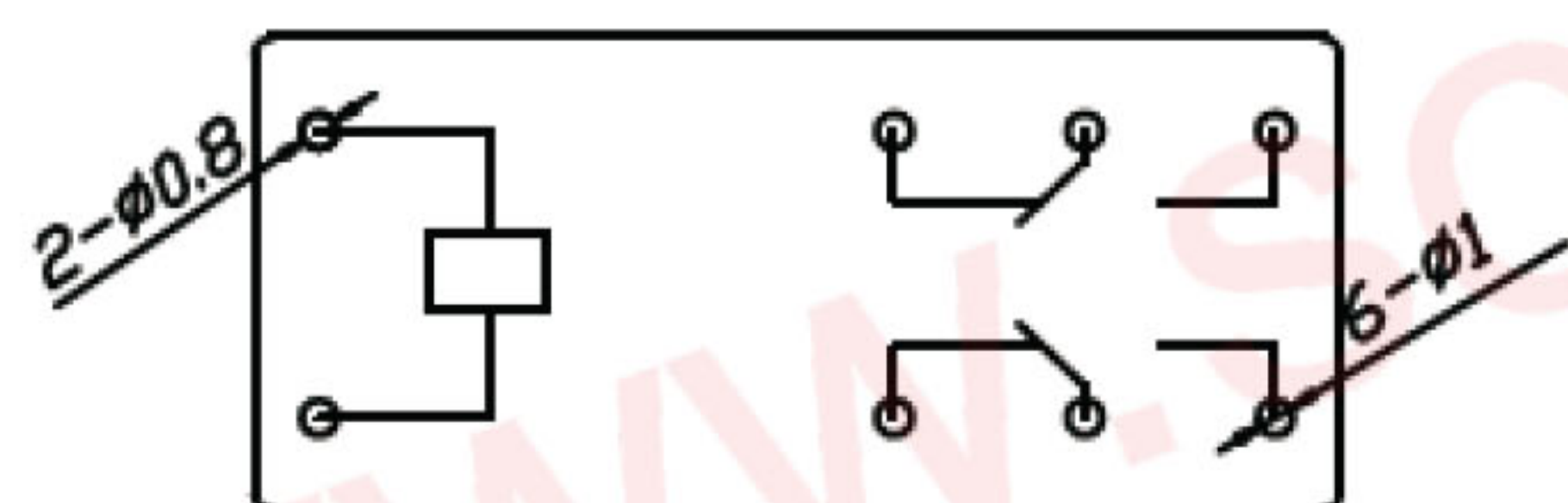
电气原理图
