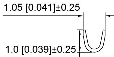
SEC:B-B
