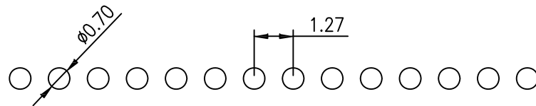
P.C.B LAYOUT
