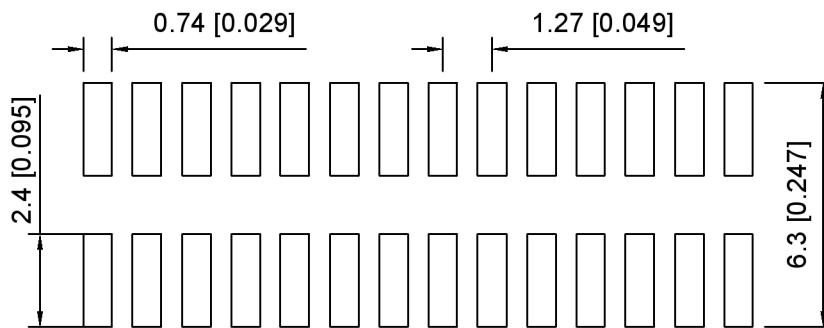
P.C.B LAYOUT
