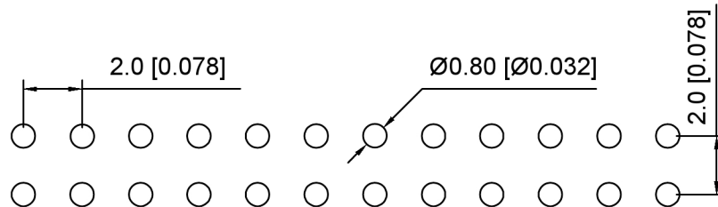
P.C.B LAYOUT
