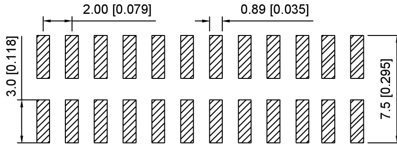
P.C.B LAYOUT
