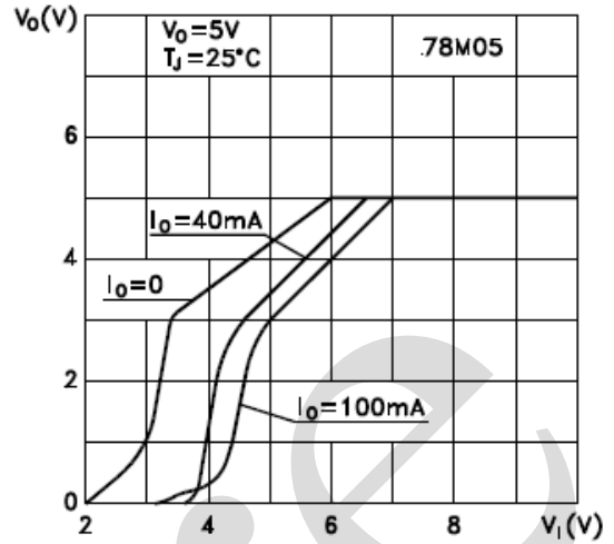
压差曲线
