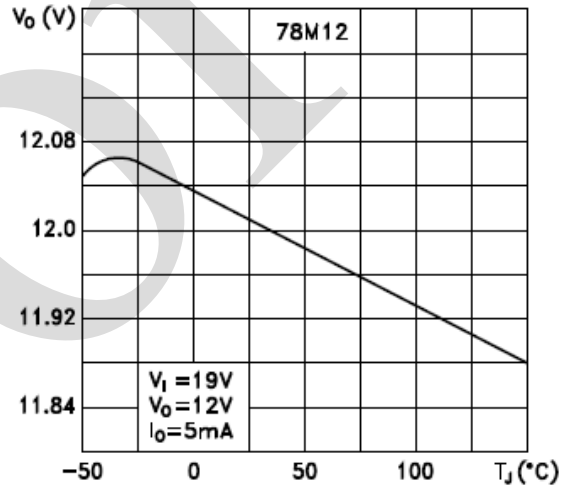
输出电压与结温的关系
