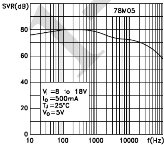
纹波抑制比
