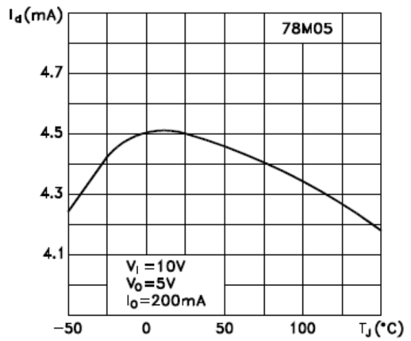
静态电流与结温的关系
